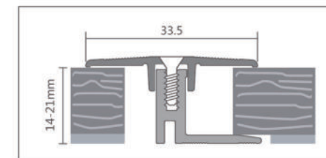
DPS 540 ♦ Suitable for 14-21mm floor ♦ 适用于14-21mm地板
