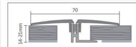
DPS 573 ♦ Suitable for 14-21mm floor ♦ 适用于14-21mm地板
