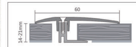
DPS 563 ♦ Suitable for 14-21mm floor ♦ 适用于14-21mm地板
