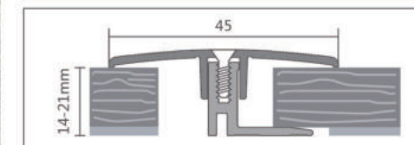
DPS 553 ♦ Suitable for 14-21mm floor ♦ 适用于14-21mm地板
